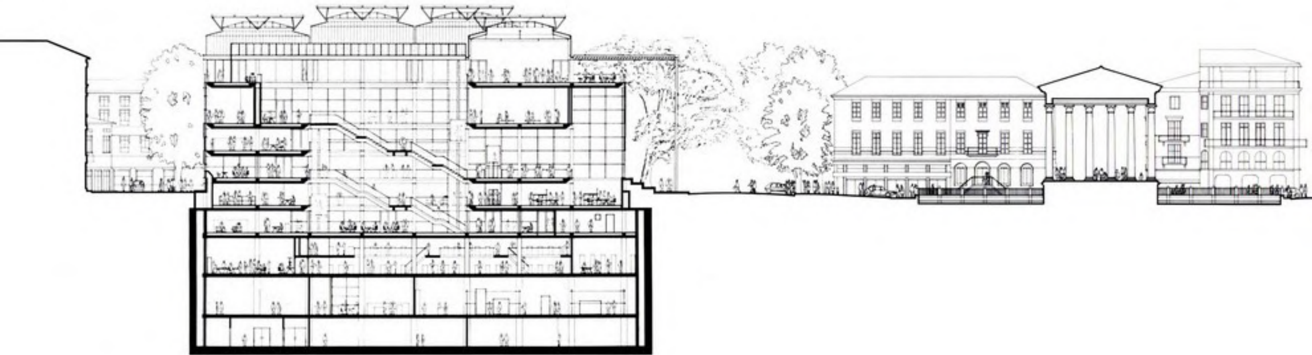
Plan en coupe Carré d'art – Maison Carré
