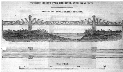
1837 Pont de Twerton (GB)
