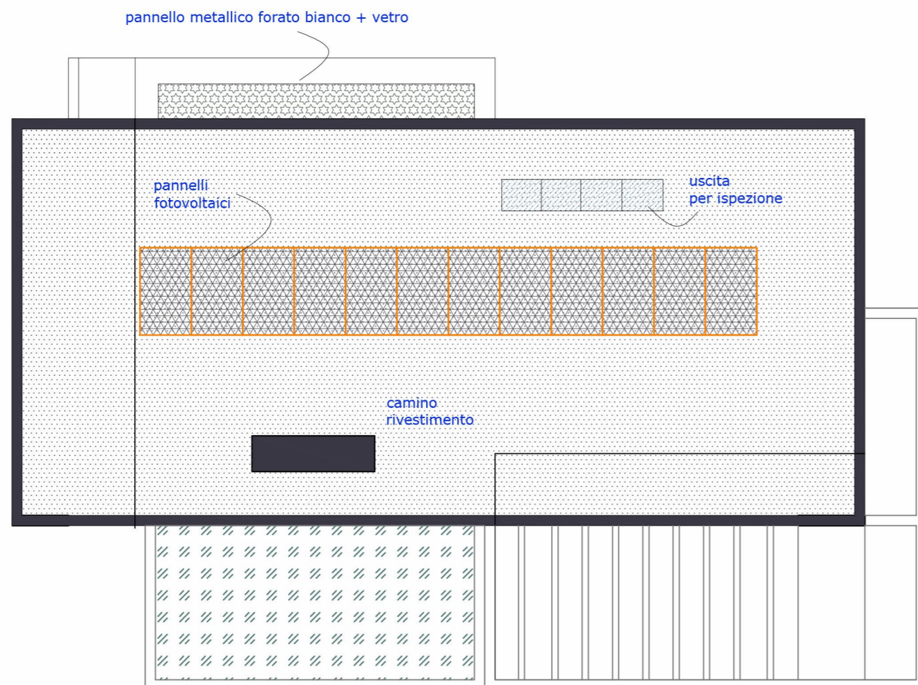
piano copertura scala 1:100
