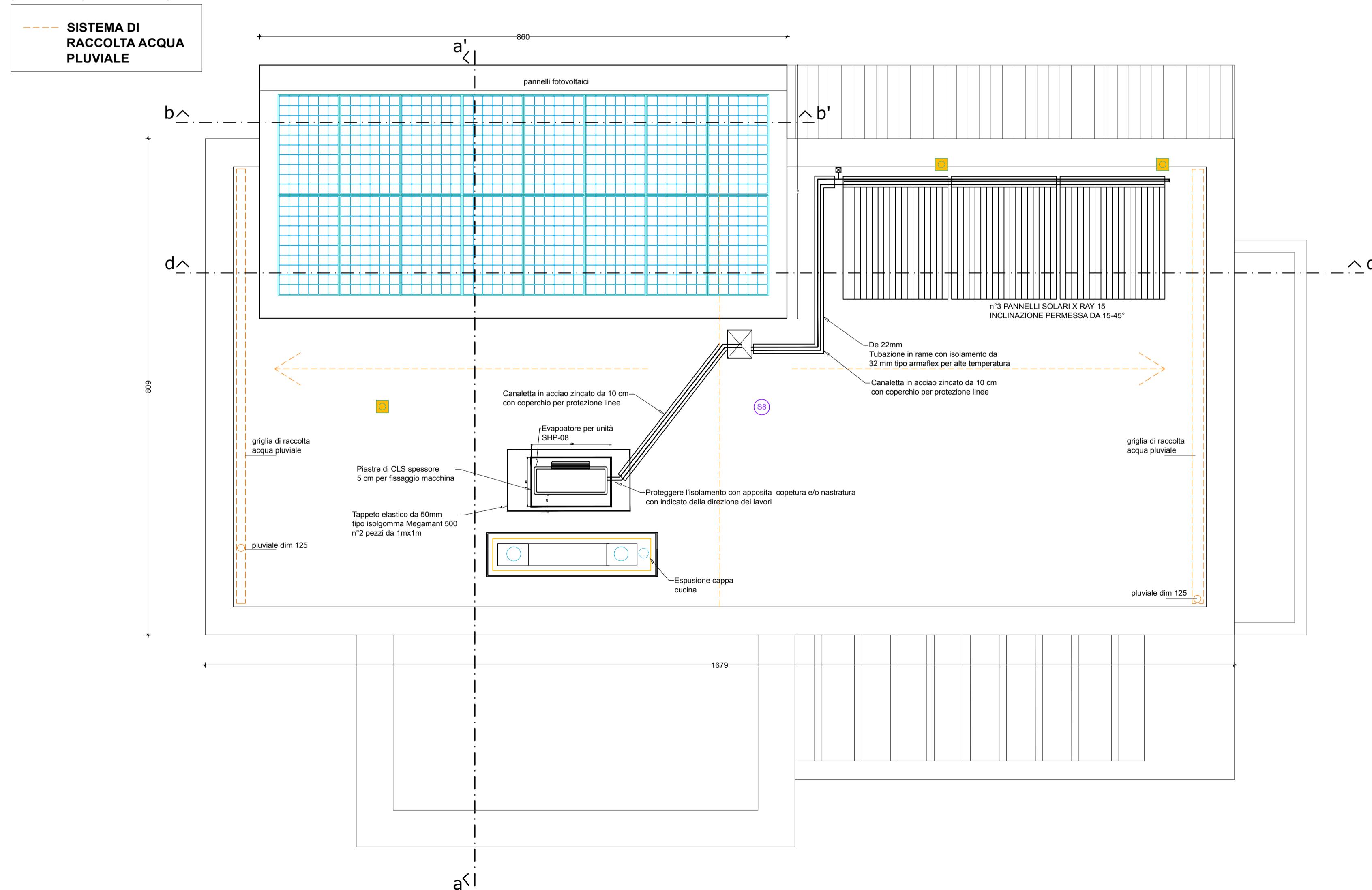
pianta piano copertura scala 1:50
