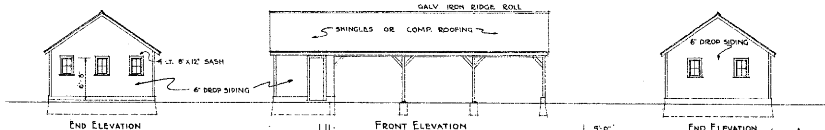
END ELEVATION
