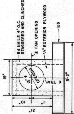
END ELEVATION
