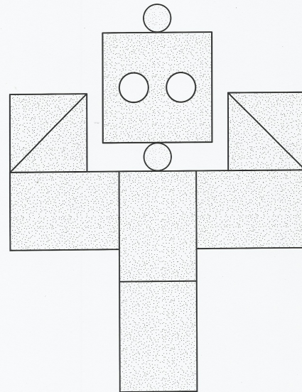
modèle 10
