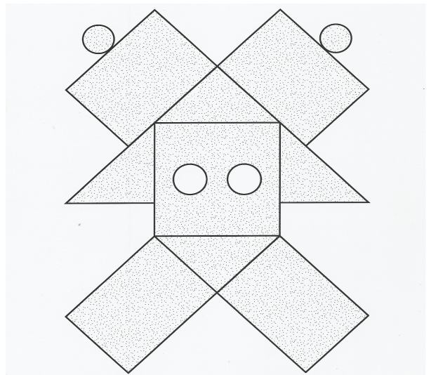
modèle 2
