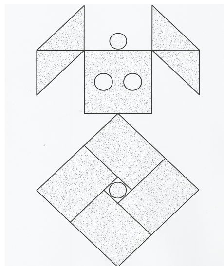
modèle 8
