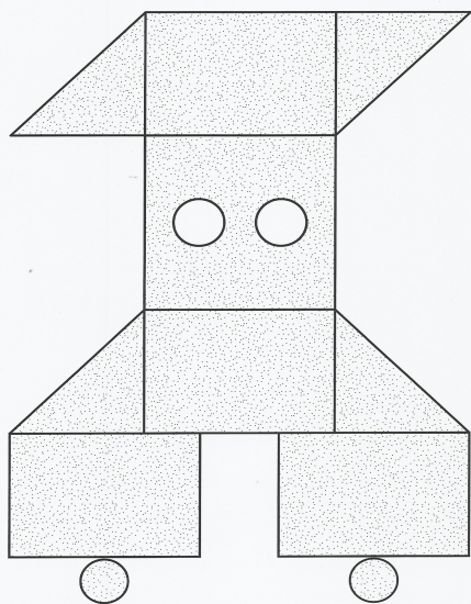
modèle 9
