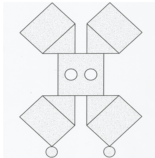
modèle 6
