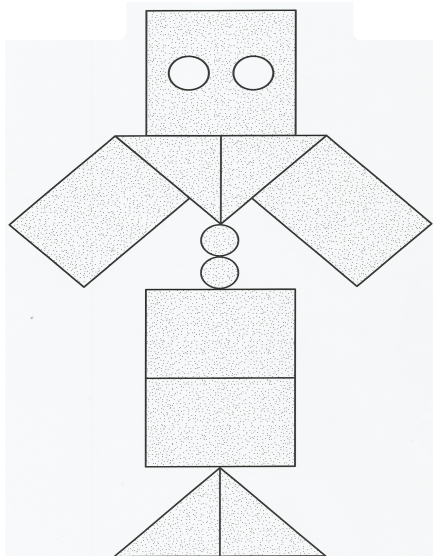
modèle 7
