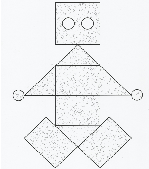
modèle 1
