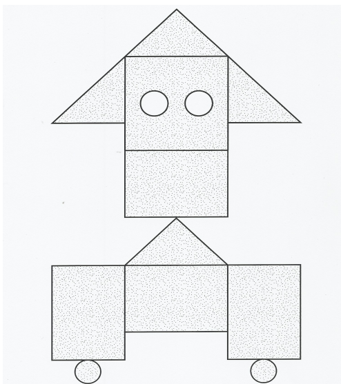
modèle 3
