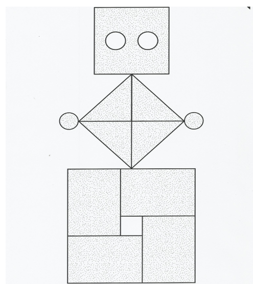
modèle 4
