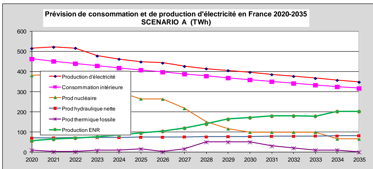
Figure 20: Prévision de consommation et de production d'électricité en France 2020-2035 (TWh) dans le scenario A.
