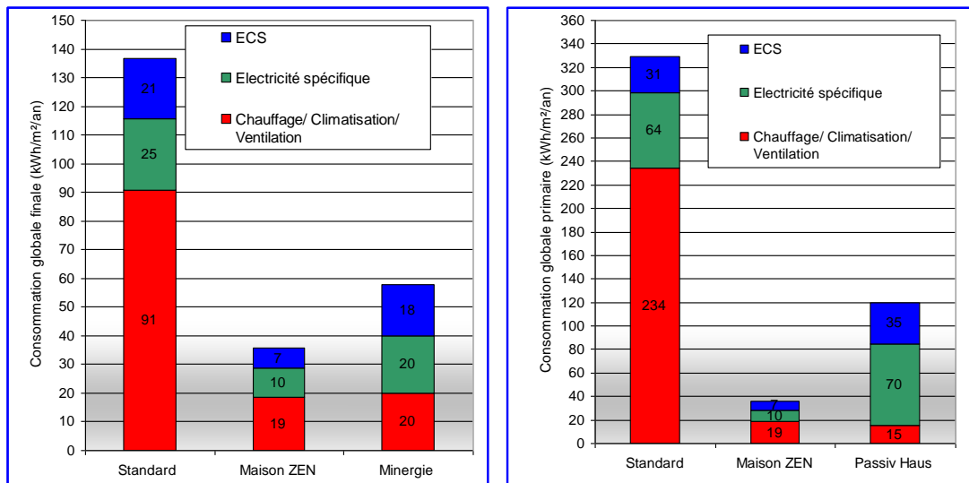
Figure 4: Comparaison construction standard, Maison ZEN (2008), Minergie et Passiv Haus
