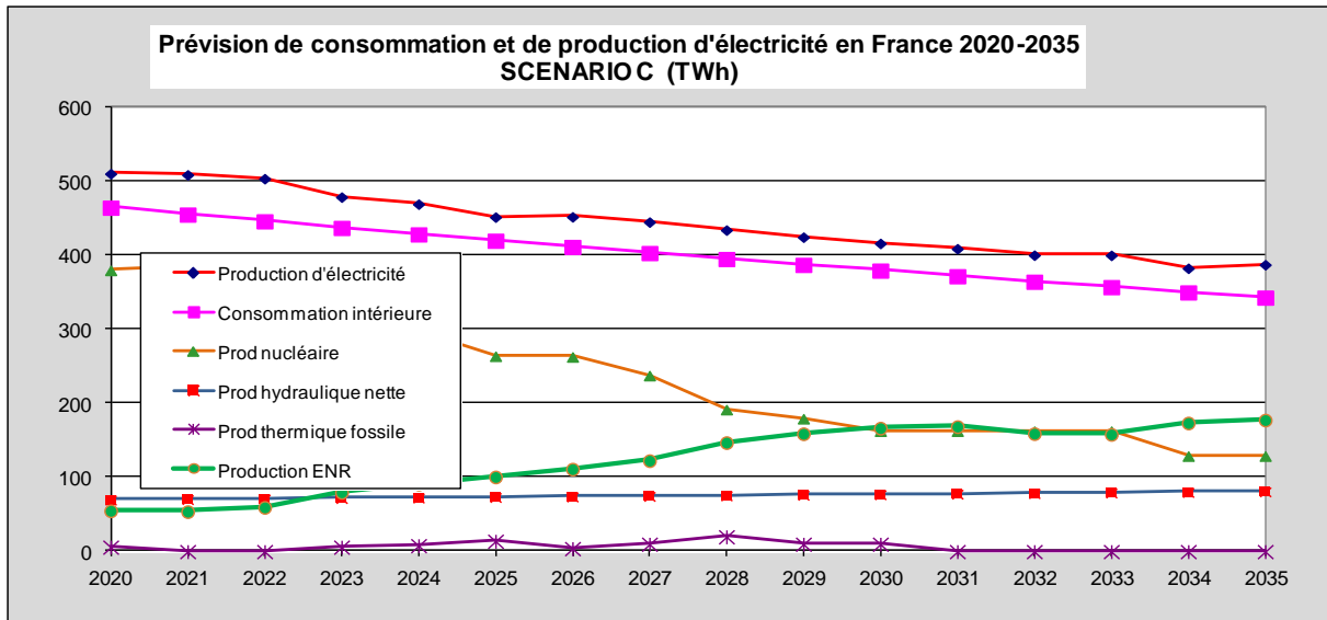
Figure 26: Prévision de consommation et de production d'électricité en France 2020-2035 (TWh) dans le scénario C.
