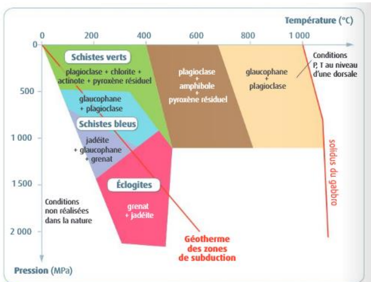
3 Diagramme de stabilité des minéraux des roches magmatiques de la lithosphère océanique. Lors du refroidissement, les gabbros de la
