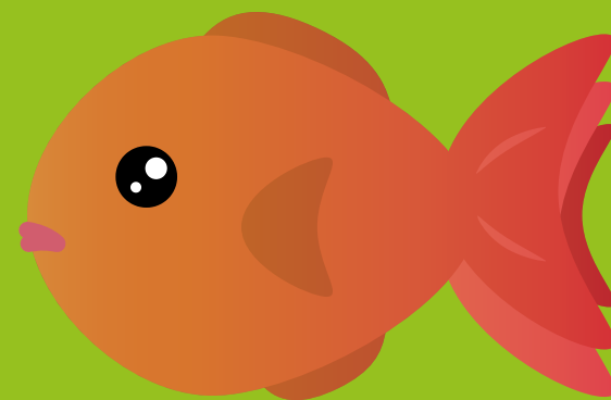
Poisson
