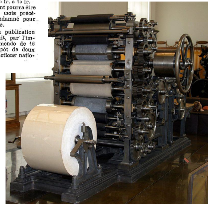
Rotative à bobine de type Marinoni (1883)
