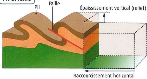
Pli et faille
