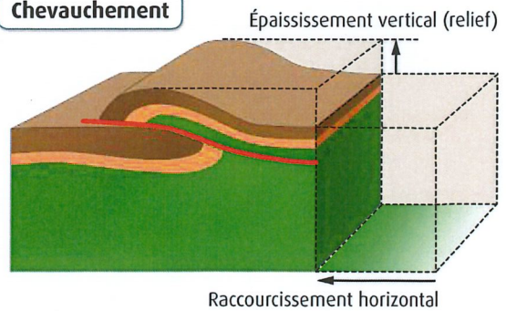
Chevauchement
