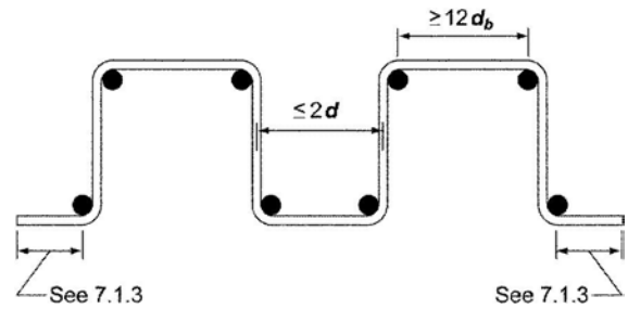
(b) multiple-leg stirrup or bar
