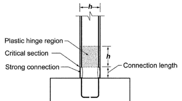
(d) Column-to-footing connection
