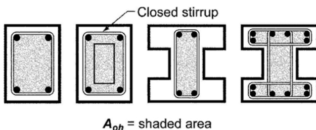
Fig. R11.5.3.6(b)—Definition of A_{oh} .
