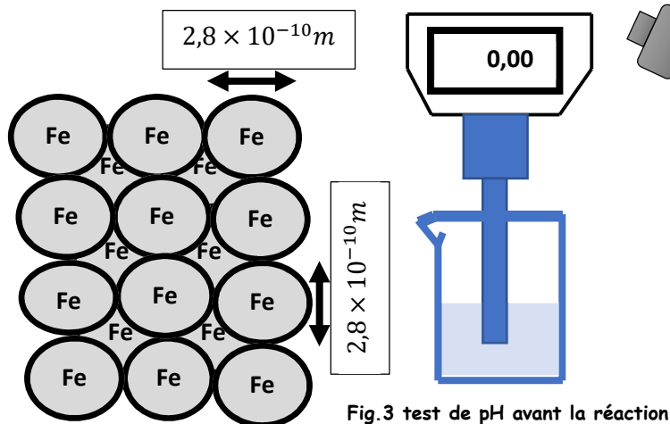
Fig.3 bis Organisation des atomes de fer
