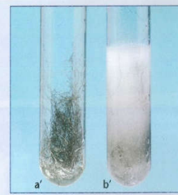
Fig.2 • Avec davantage de laine de fer.
