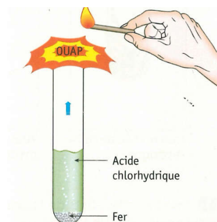
Fig.5 • Action de l'acide chlorhydrique sur le fer.
