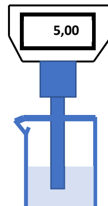
Fig.6 Test de pH après quelques jours
