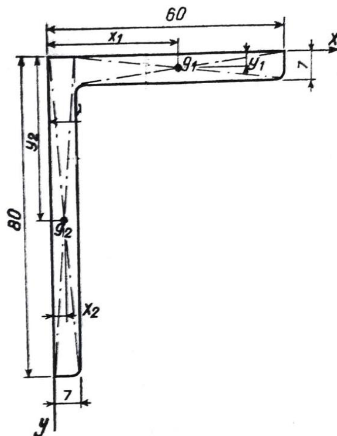
FIG. 1-4. — Ailes de 7 mm d'épaisseur.
