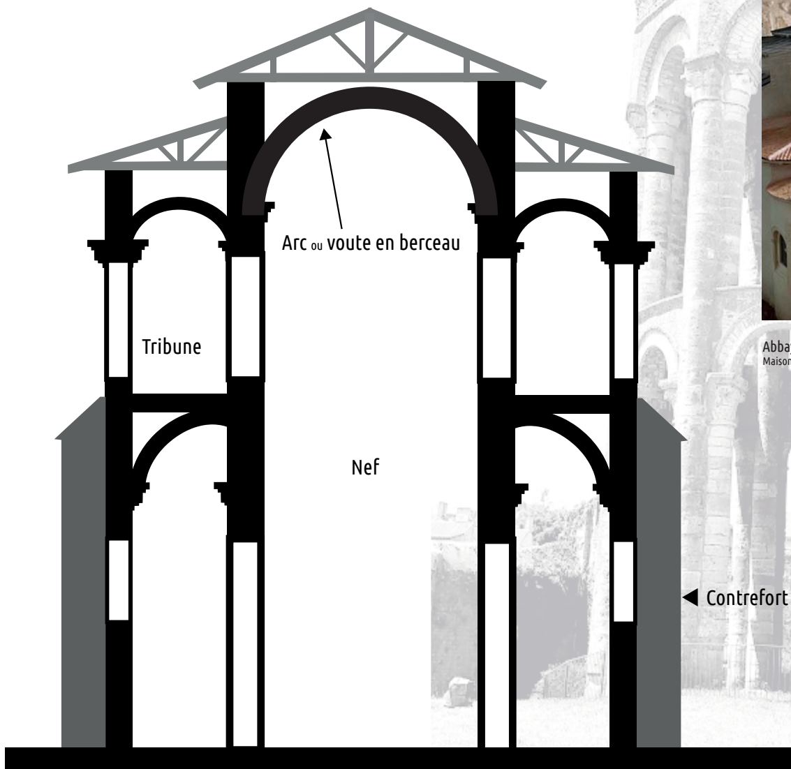
Coupe de la nef d'une église Romane
