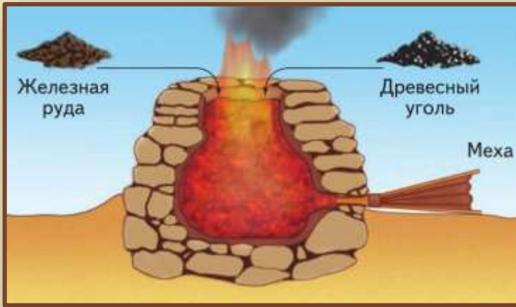
Печь-домница
