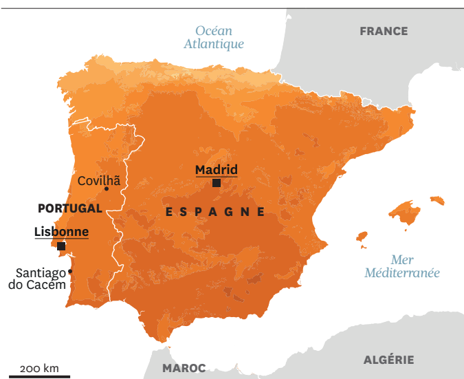
Potentiel de puissance photovoltaïque (1994-2018) (moyenne des totaux journaliers en kWh/kWp sur un an)*
