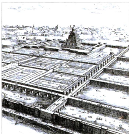
План древнего Вавилона. Реконструкция.
