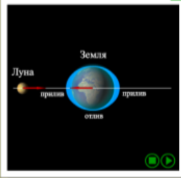
ОБРАЗОВАНИЕ ПРИЛИВОВ
