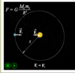
ВСЕМИРНОЕ ТЯГОТЕНИЕ
