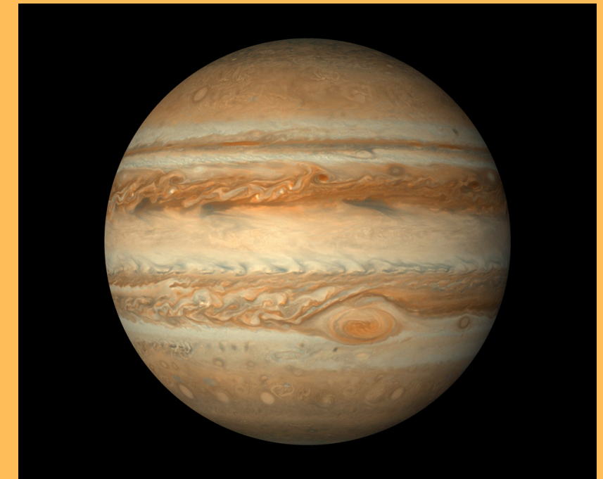
Jupiter
