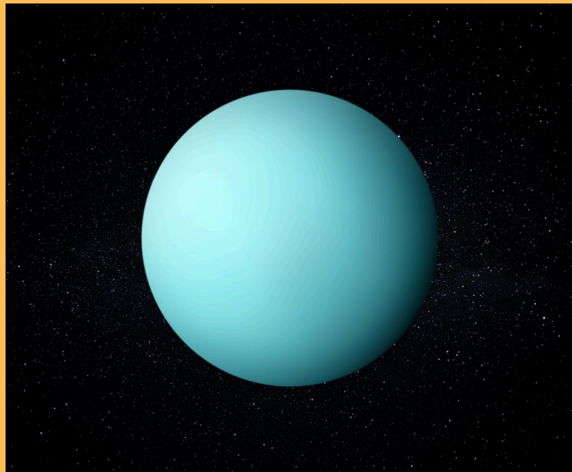
Uranus
