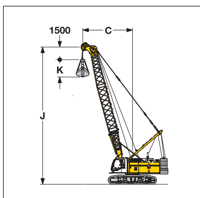
Portate in tonnellate (t) per lunghezze del braccio da 14 m a 29 m Zavorra 26.3 t
