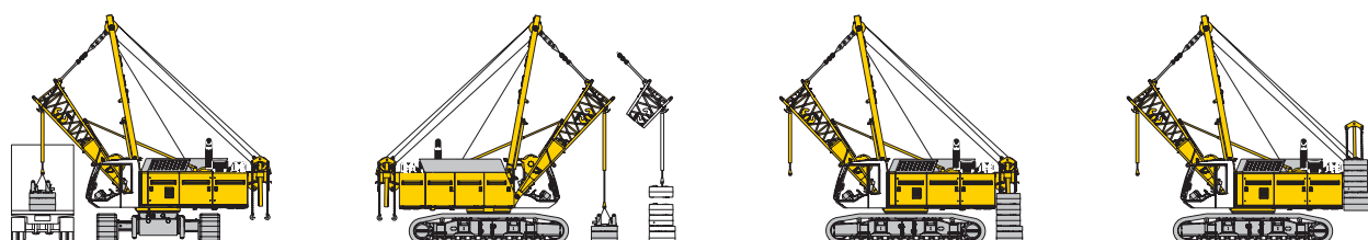
Scaricamento ed assemblaggio della zavorra
