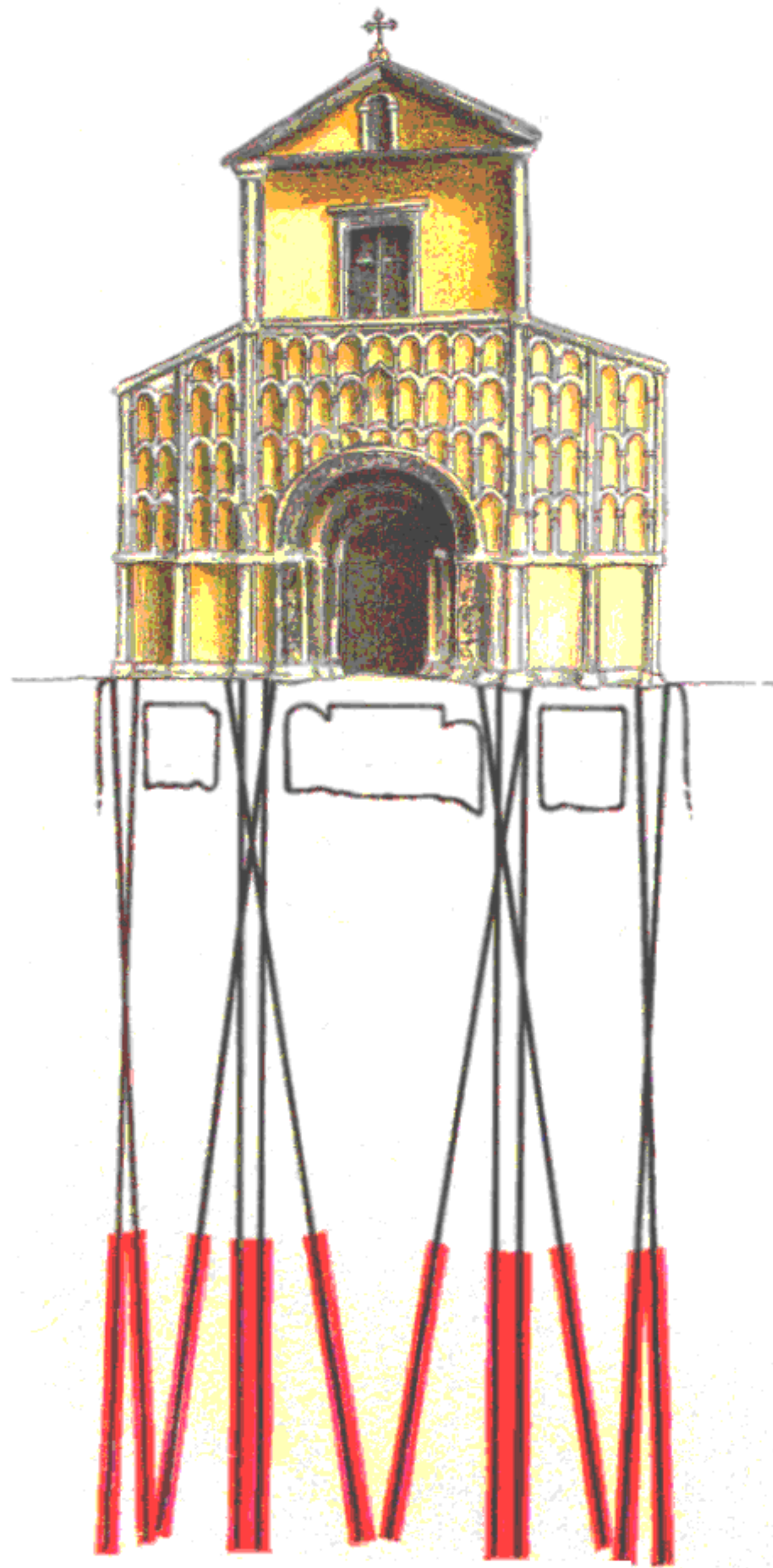
Stabilizzazioni di fondazioni
