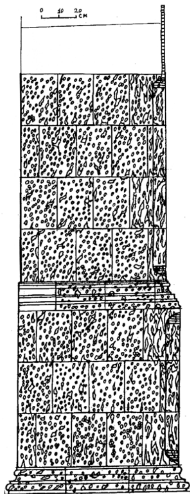
Мал. 18. Частковая рэканструкцыя магчымага выгляду паўднёвага фасада печы з памяшкання № 2 корпуса «А».
