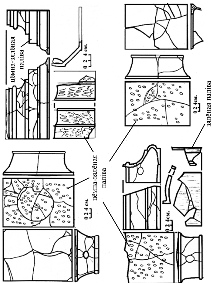
Мал. 9. Кафля другаснага ўжытку з падмурка печы памяшкання № 2 корпуса «А».
