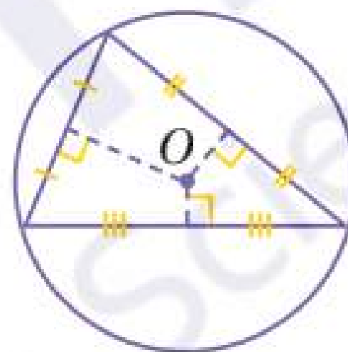
Описане коло навколо трикутника
