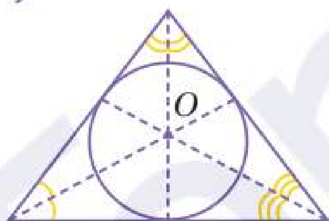
Вписане коло в трикутник
